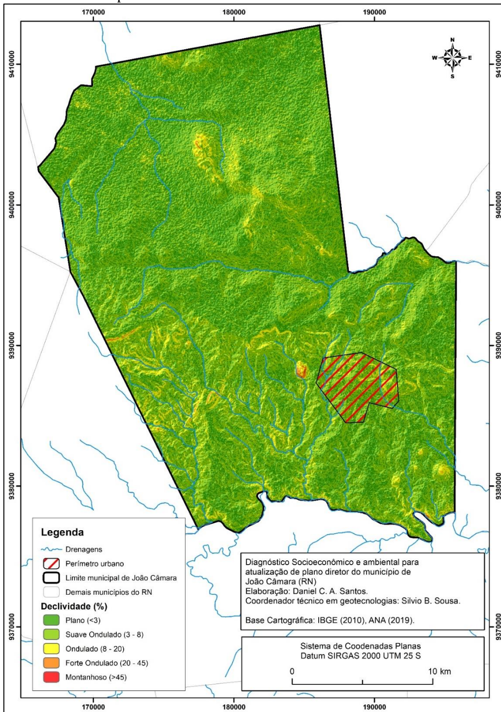
Mapa 8 - João Câmara: Percentual de declividade.
