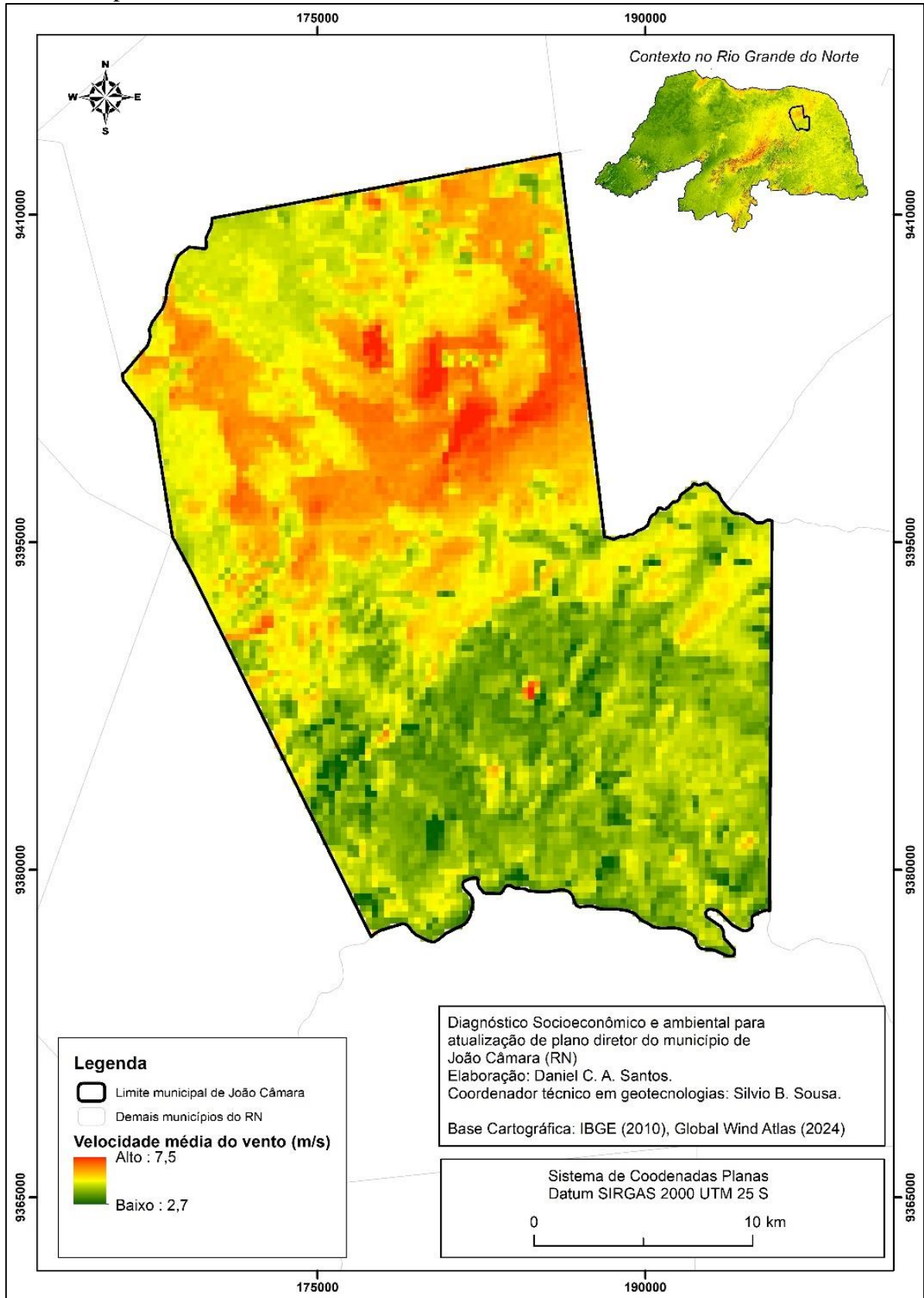
Mapa 13 - Velocidade média do vento a 10 metros de altura, em escala anual.
