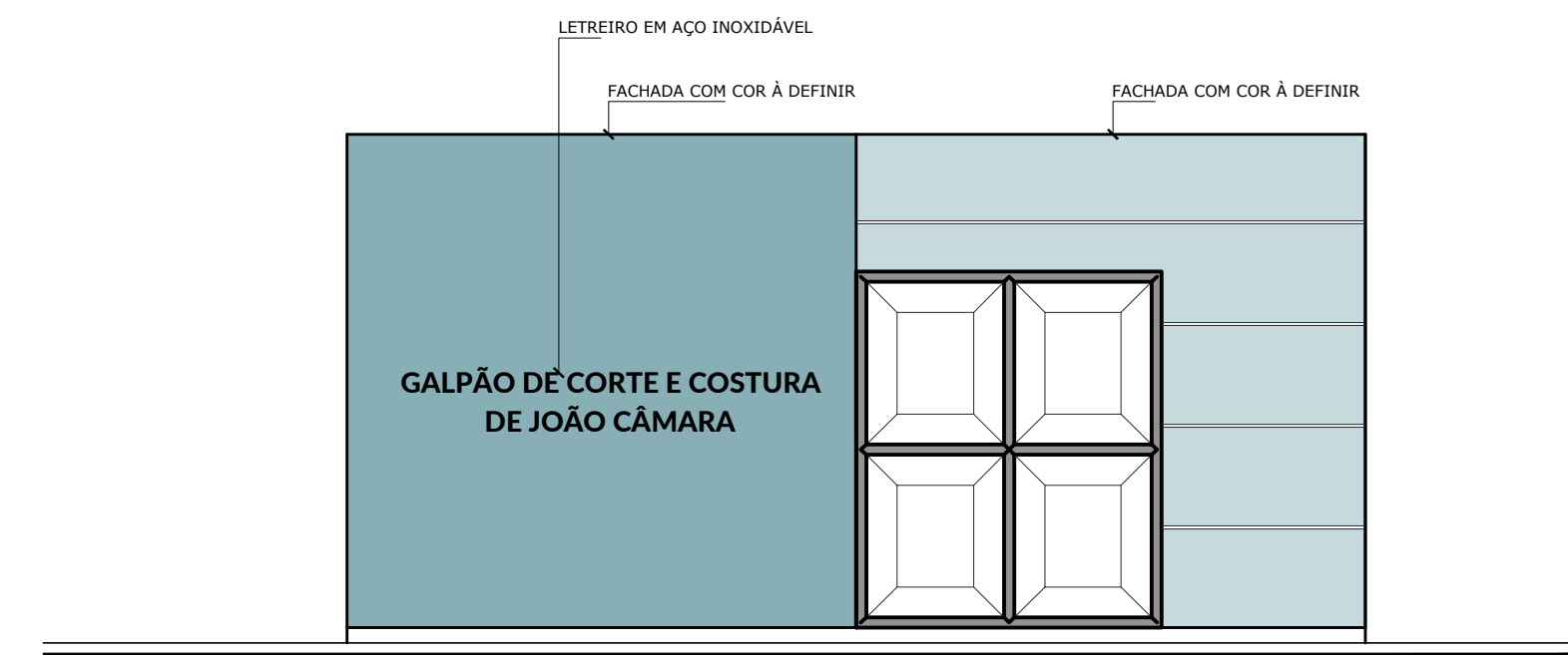
FACHADA FRONTAL ESCALA ..... 1 : 75
